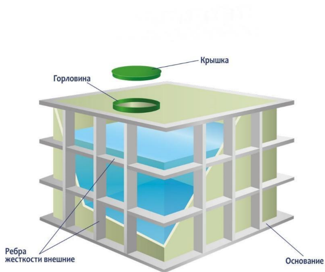
Рисунок 10. ГРИНЛОС Емкость прямоугольная наземная в металлическом каркасе в разрезе
