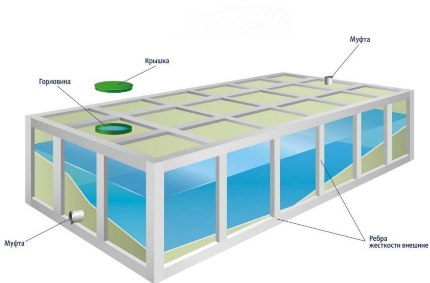
Рисунок 12. ГРИНЛОС Емкость прямоугольная наземная в металлическом каркасе в разрезе
